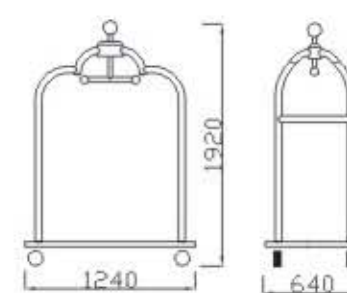
92.2010A Dimension
