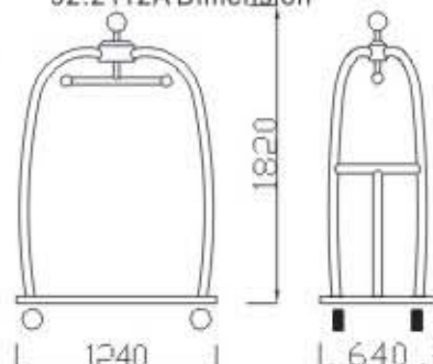
92.2112A Dimension
