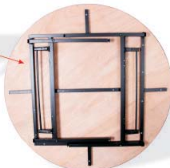
99.1530R背面
