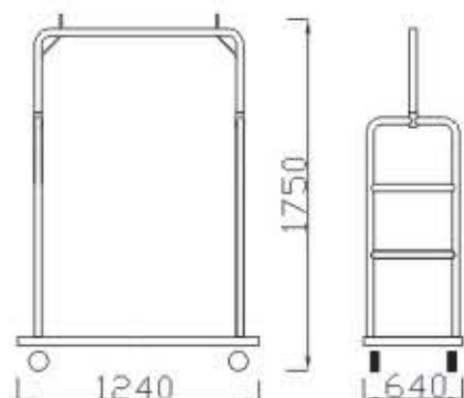
90.2007A Dimension
